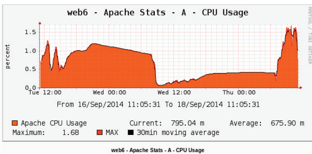
Software de Generación de Gráficos Cacti
